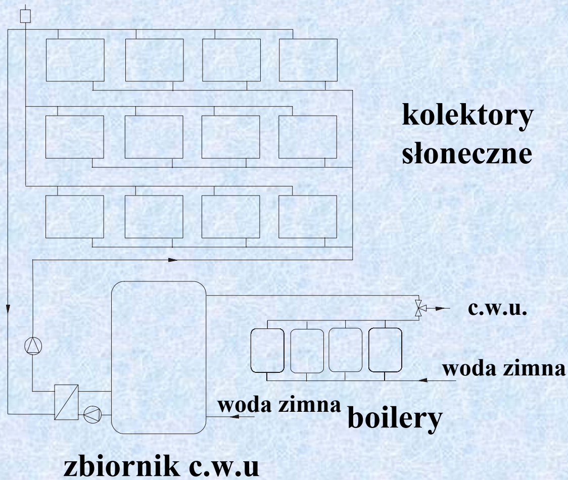
Schemat ogólny kolektora słonecznego
